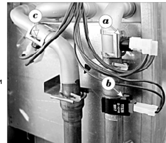
Рис. 21 - Датчик температуры
