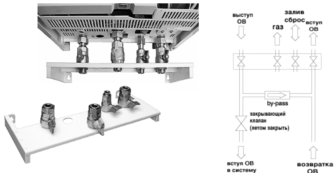
Рис. 7 – Присоединительный комплект
