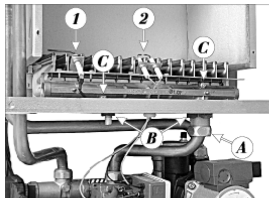
Рис. 17 – Монтаж горелки
