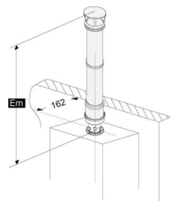
Рис. 10 Пример вертикальной трассы коаксиальной трубы – исполнение C 32 (ЧСН ЕН 483)
