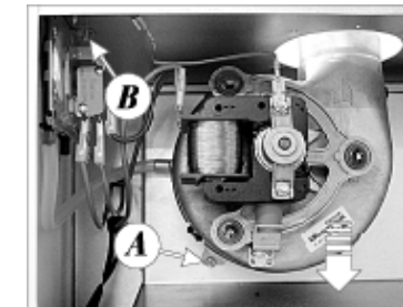
Рис. 18 – Монтаж вентилятора
