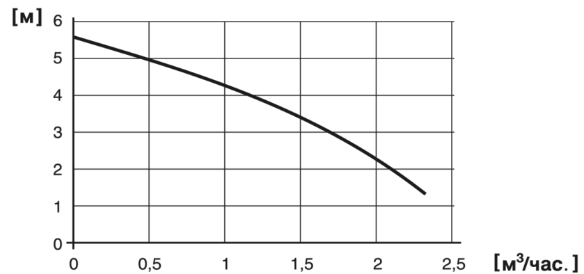
Рис. 5 – Характеристика насоса
