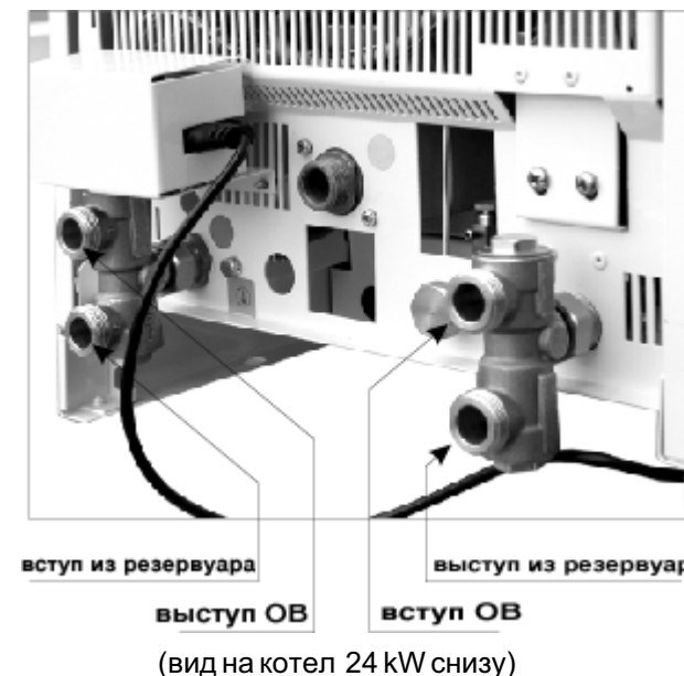
Рис. 15 – Присоединение комплекта для работы с внешним резервуаром
