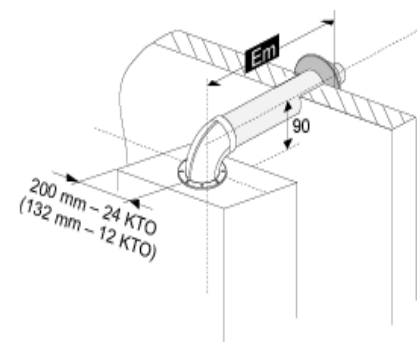
Рис. 9 Пример горизонтальной трассы коаксиальной трубы – исполнение C 12 (ЧСН ЕН 483)
