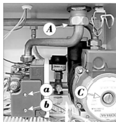
Рис. 20 – Газовый вентиль
